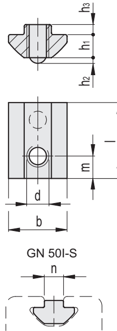
GN 50I-S-SZ
