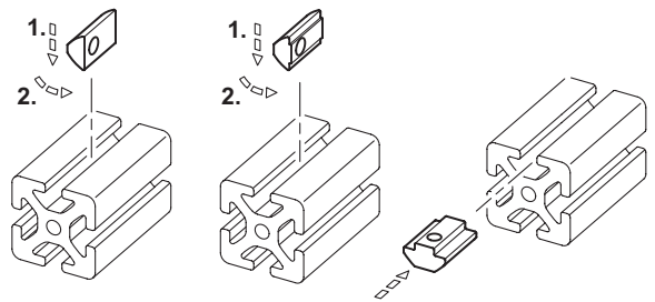
GN 50I-N
